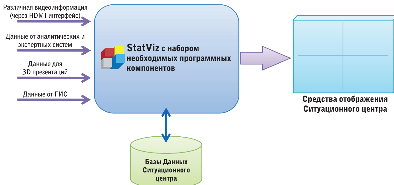
Функциональная схема «Модуля интеграции и визуализации информации Ситуационного центра на основе StatViz»
